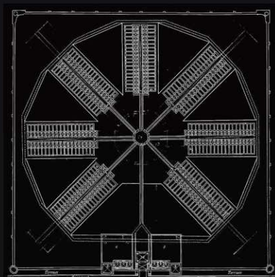
Plan du pénitencier de Pennsylvanie, 1830
